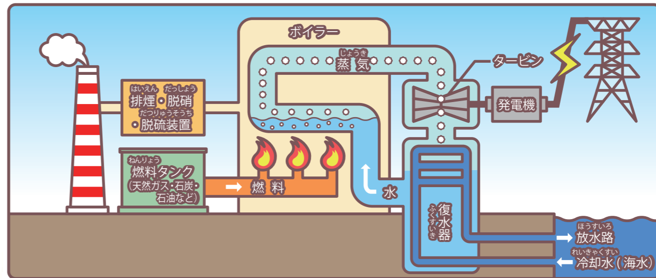
せき たん か り ゅ く は つ でん 石炭火力発電のしくみ
